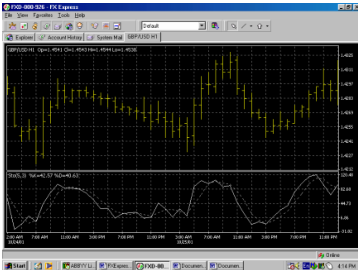
Рис. 5.40. Пример стохастика
