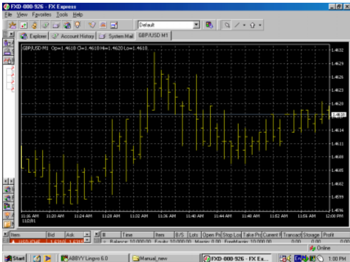
Рис. 5.5. Пример гистограммы
